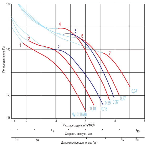
ВКП-...-5-...x1000-...
