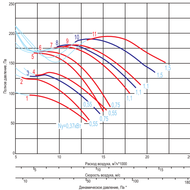
...-7,1-...x1000-...
