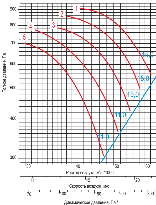
ВО 25-188-10
