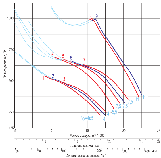
ВКП-...-6,3-...x1500-...
