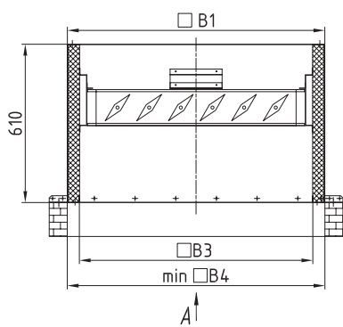
Стакан СТКВ-М
