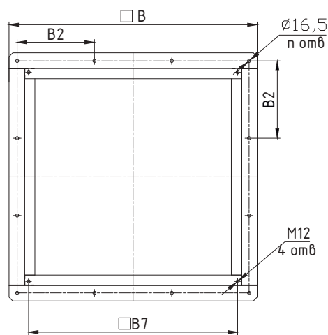
Стакан СТКУ-М
