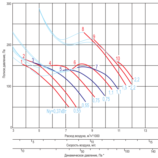
ВКП-...-5,6-...x1500-...
