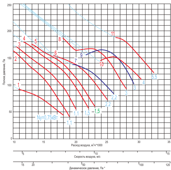
ВКП-...-10-...x750-...
