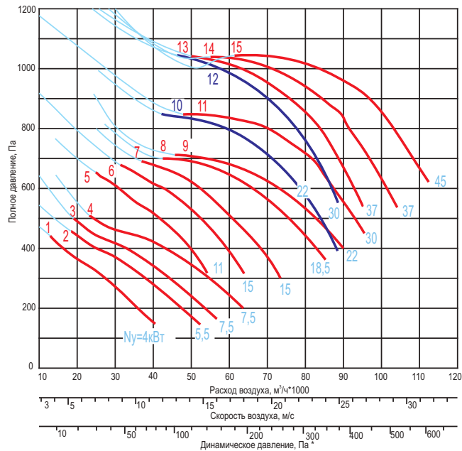
...-11,2-...x1500-...
