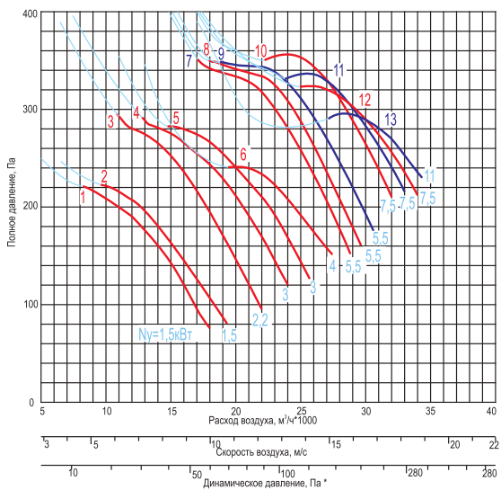
ВКП-...-9-...x1000-...
