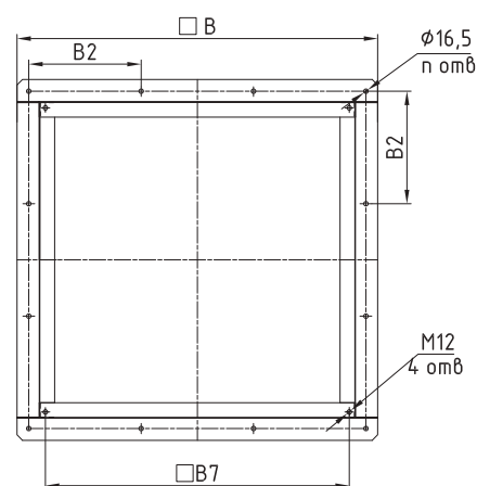
Стакан СТКУ-П
