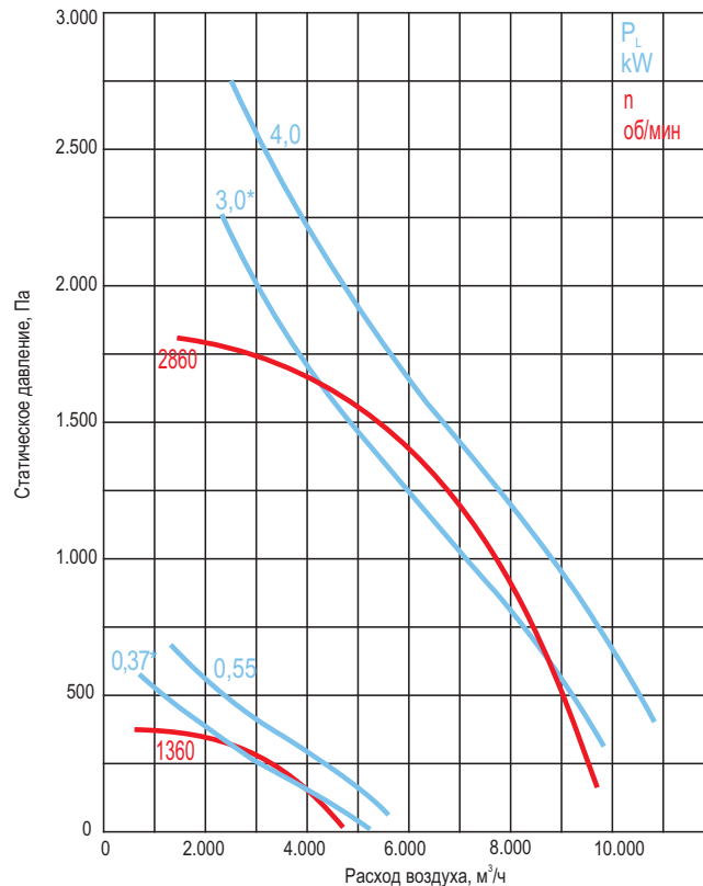
ВКР-4-ДУ-Ф-...
