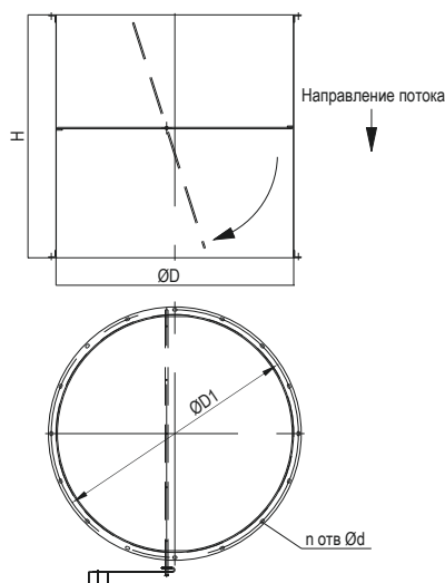
Технические характеристики клапанов обратных для вентиляторов ВО
