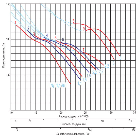
ВКП-...-10-...x750-...
