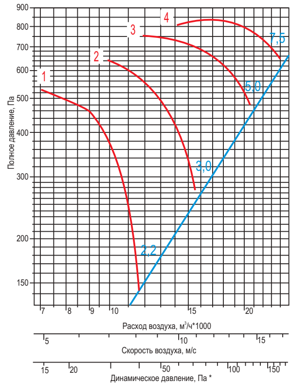
ВО 30-160-071
