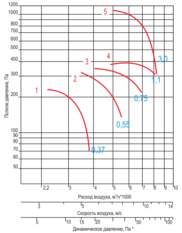
ВО 30-160-050
