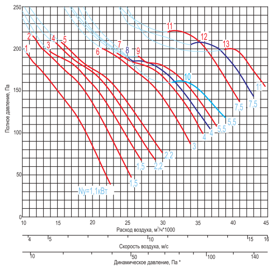
ВКП-...-10-...x1000-...
