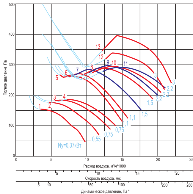
...-6,3-...x1500-...
