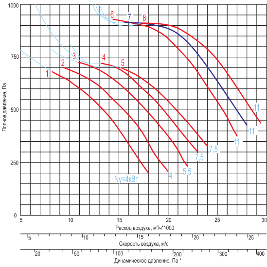
ВКП-...-6,3-...x3000-...
