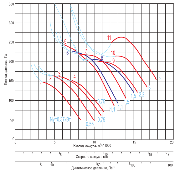
ВКП-...-6,3-...x1500-...
