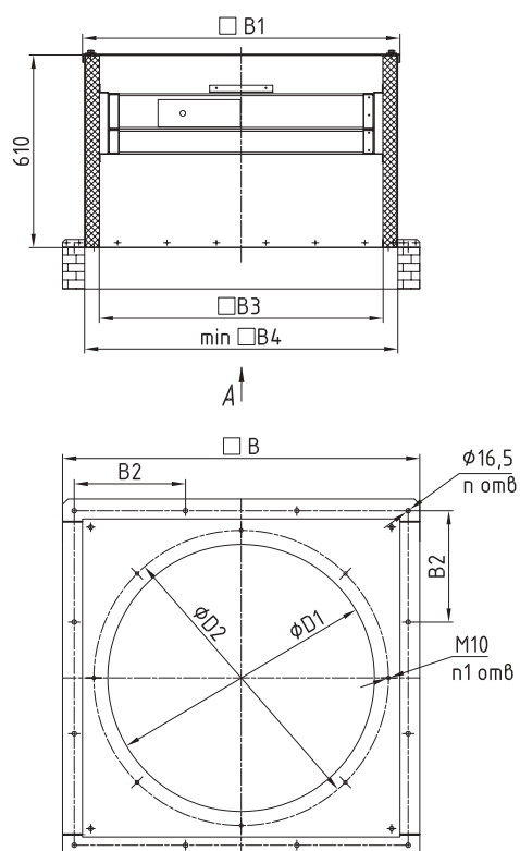
Стакан STKV-P
