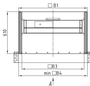
Стакан СТКУ-М
