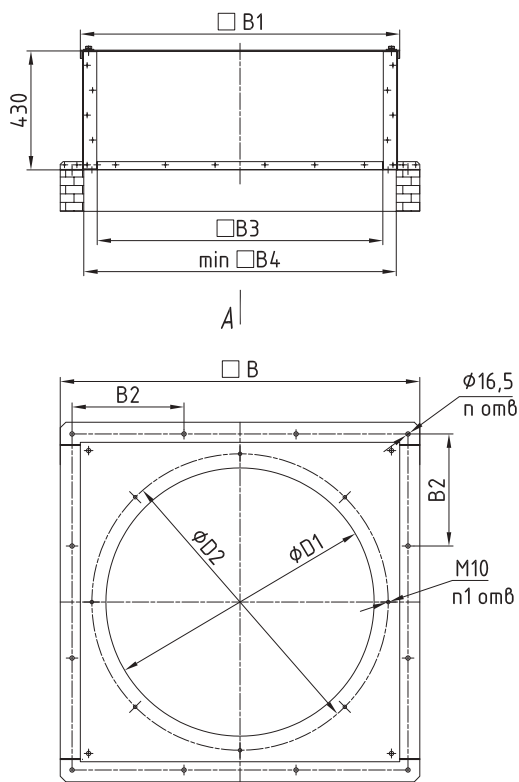
Стакан STKB-M
