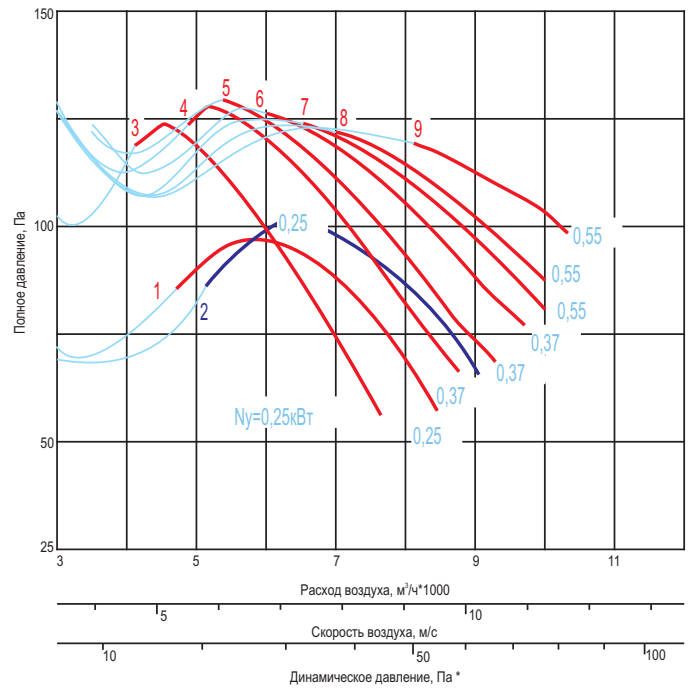
...-5,6-...x1000-...
