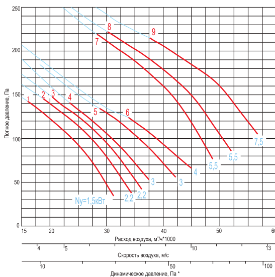
ВКП-...-12,5-...x750-...
