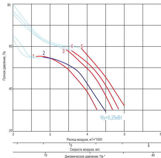
ВКП-...-5-...x1000-...
