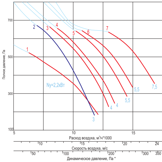
ВКП-...-5-...x3000-...
