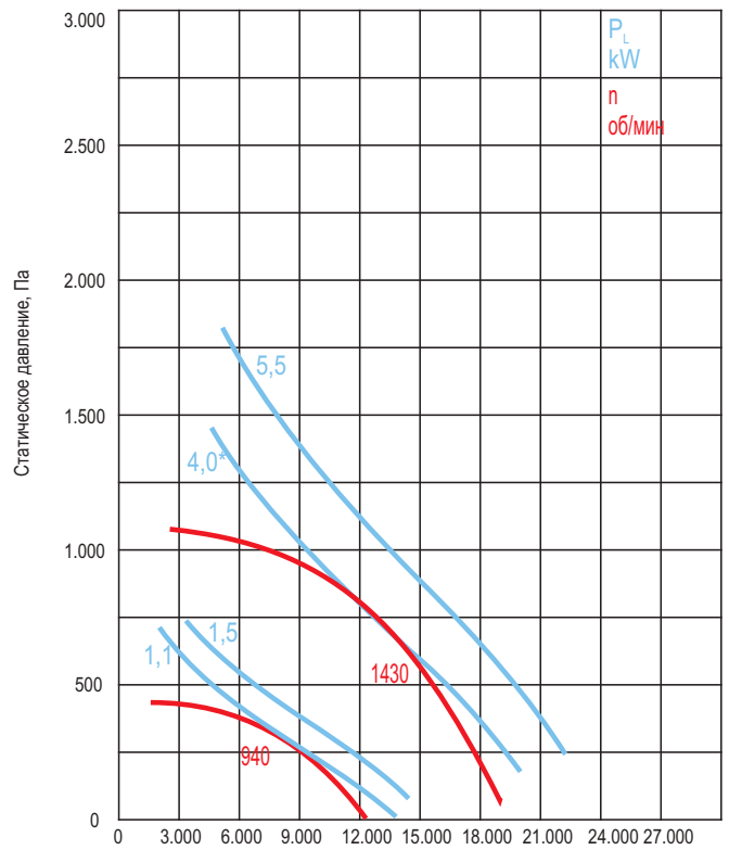
ВКР-6,3-ДУ-Ф-...
