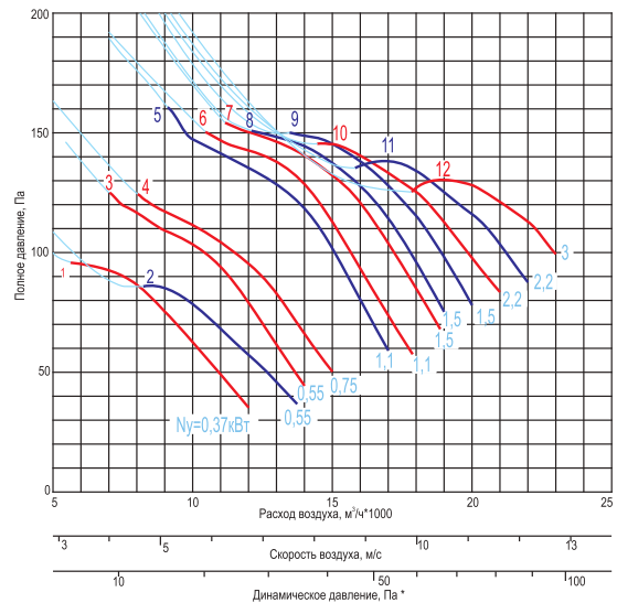
ВКП-...-8-...x1000-...
