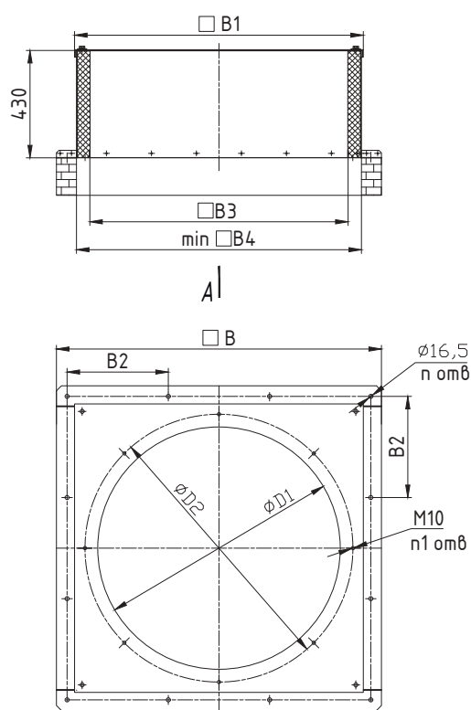
Стакан STKV-M
