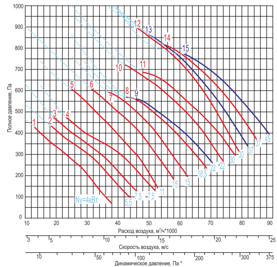
ВКП-...-11,2-...x1500-...
