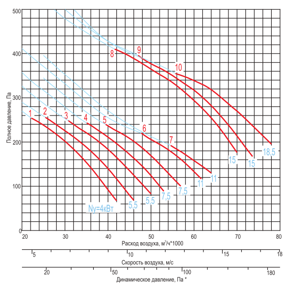
ВКП-...-12,5-...x1000-...
