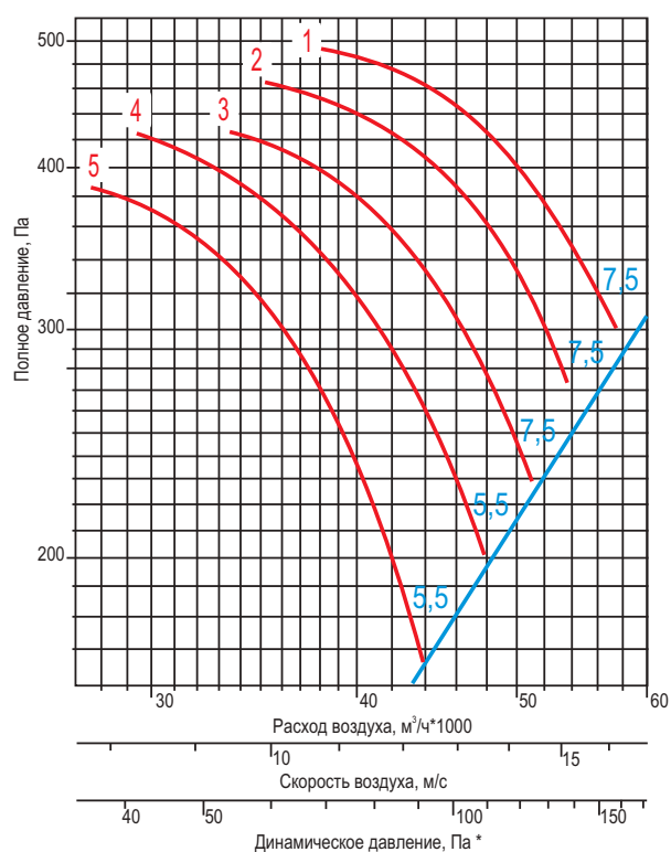
ВО 25-188-11,2
