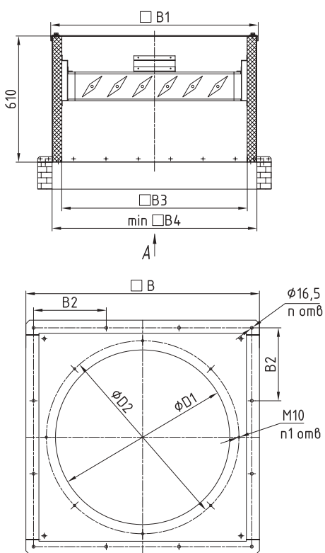
Стакан STKV-K
