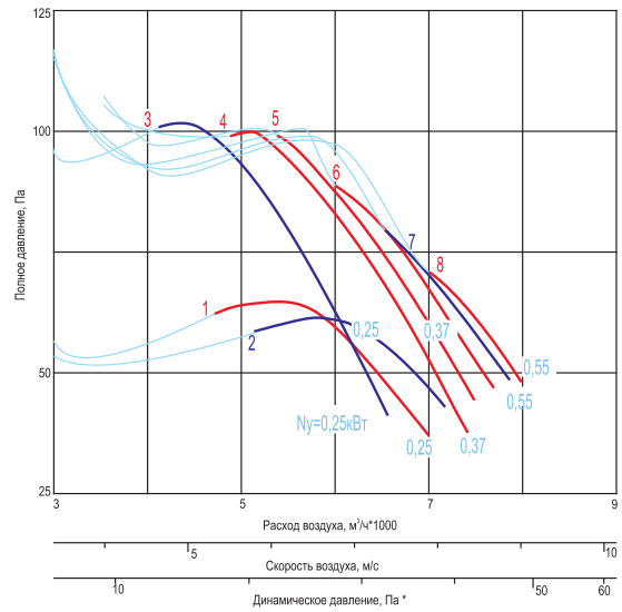
ВКП-...-5,6-...x1000-...
