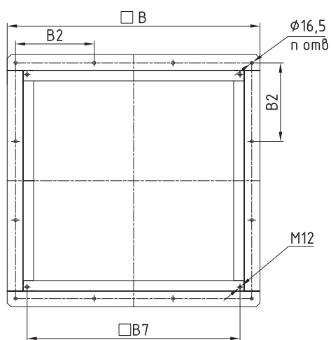
Стакан СТКВ-М
