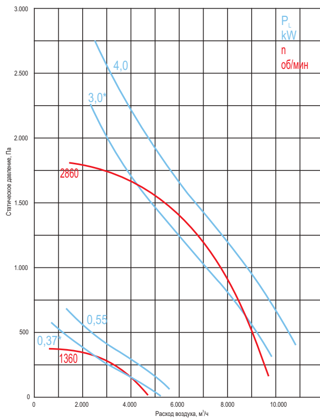
ВКР-4-ДУ-В-...
