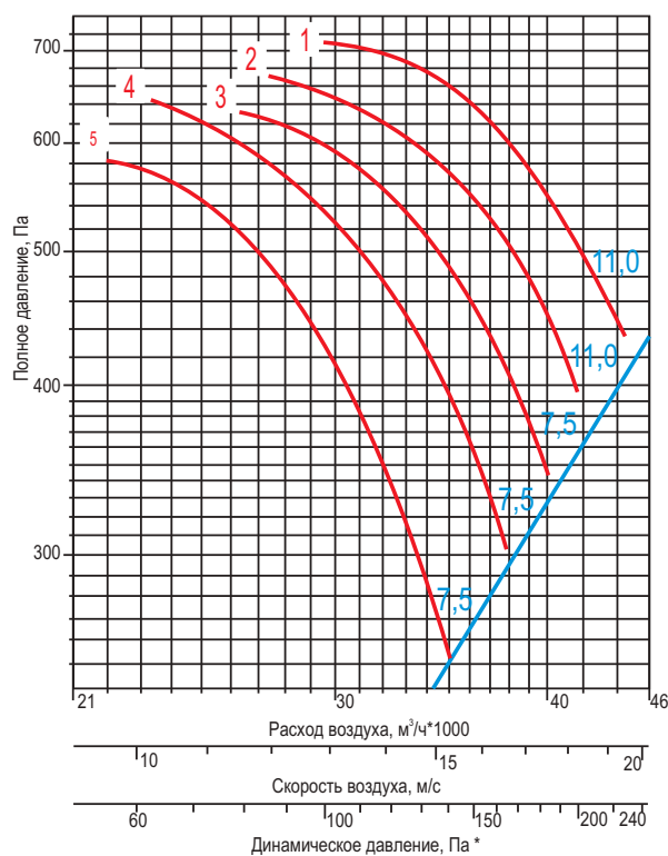
ВО 25-188-9
