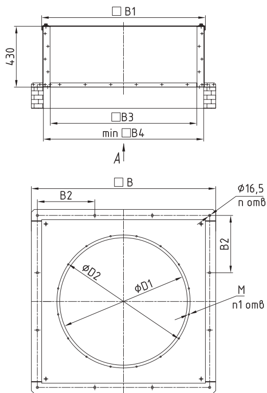
Стакан СТКВ-М
