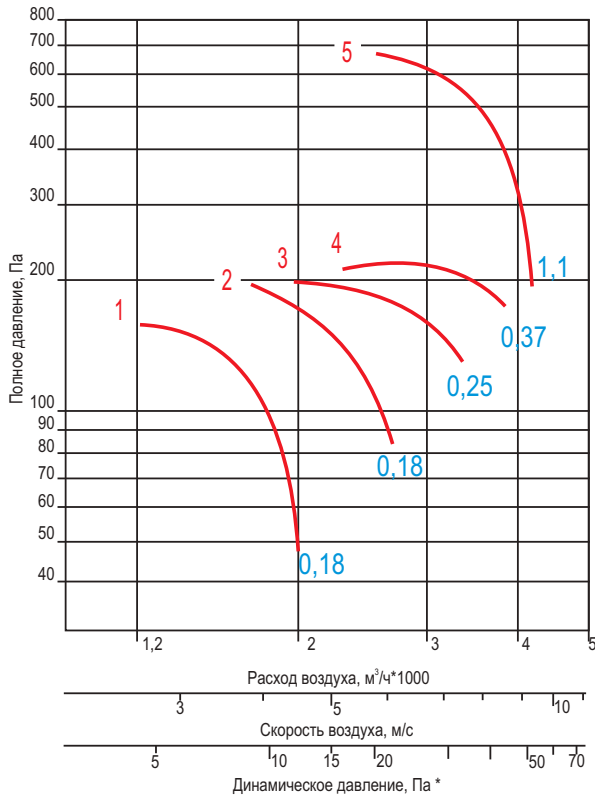
ВО 30-160-040
