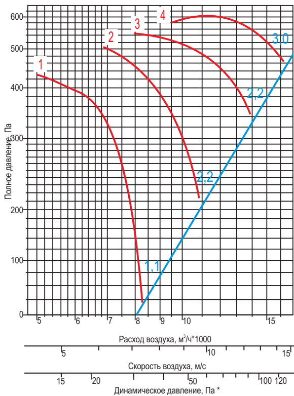
ВО 30-160-063
