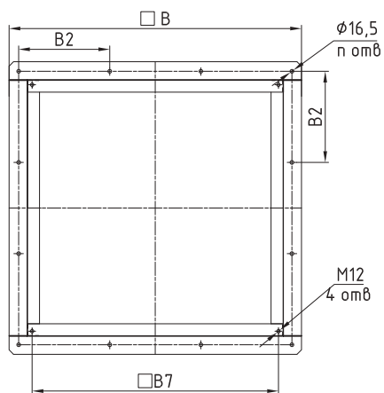
Стакан СТКУ-К
