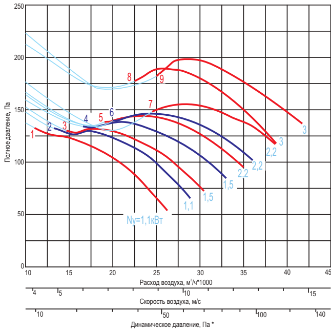
...-10-...x750-...
