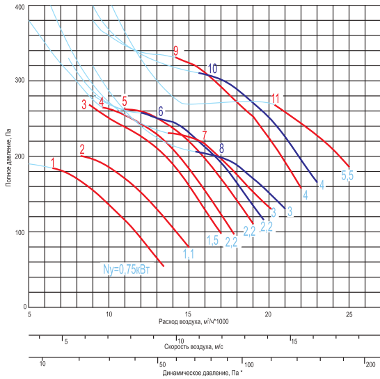
ВКП-...-8-...x750-...
