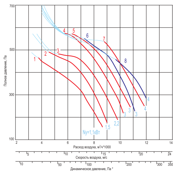
ВКП-...-5-...x1500-...
