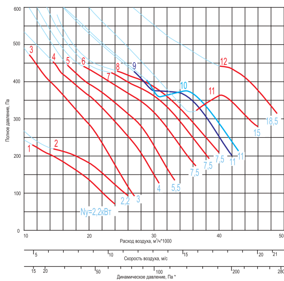
ВКП-...-10-...x1000-...
