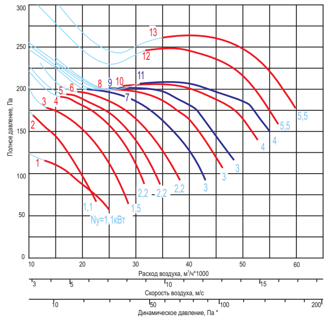
...-11,2-...x750-...
