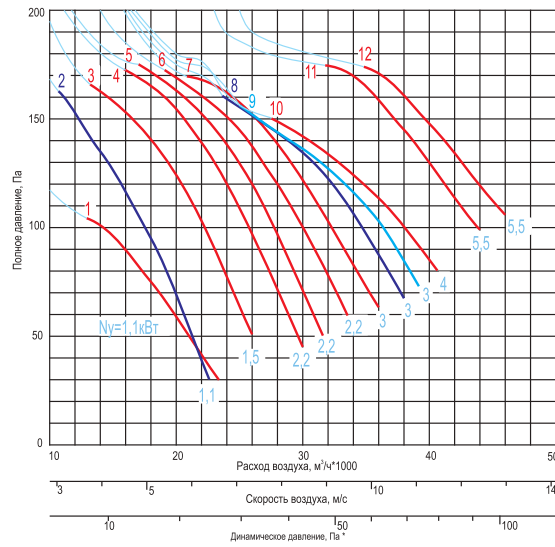
ВКП-...-11,2-...x750-...
