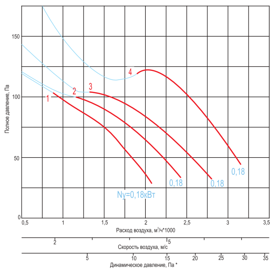
ВКП-...-4-...x1500-...
