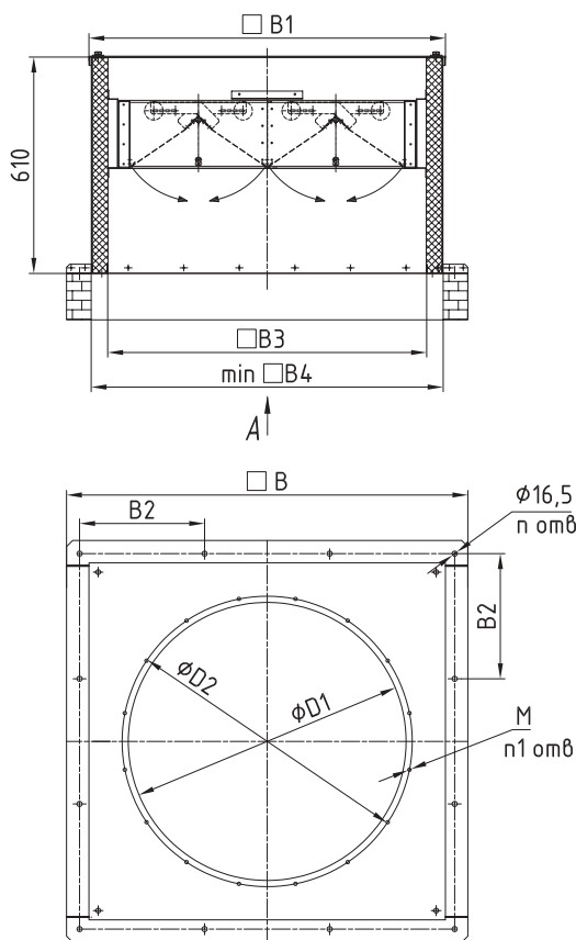
Стакан СТКУ-П - приток
