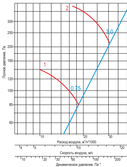
ВО 12-303-8
