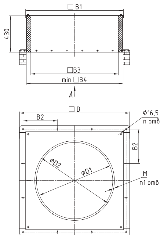
Стакан СТКУ-М
