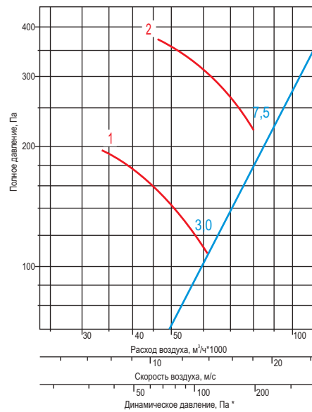
ВО 12-303-12,5
