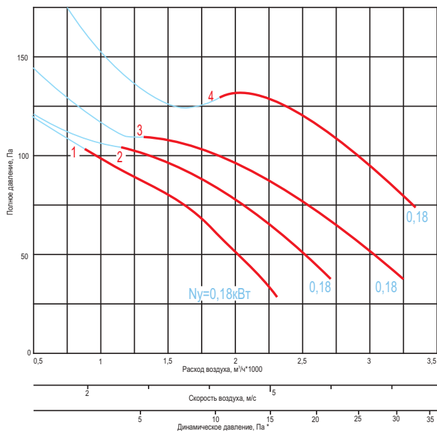
...-4-...x1500-...
