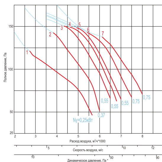
ВКП-...-5-...x1500-...
