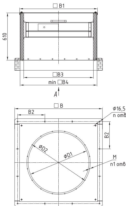
Стакан СТКУ-П/СТКУ-К
