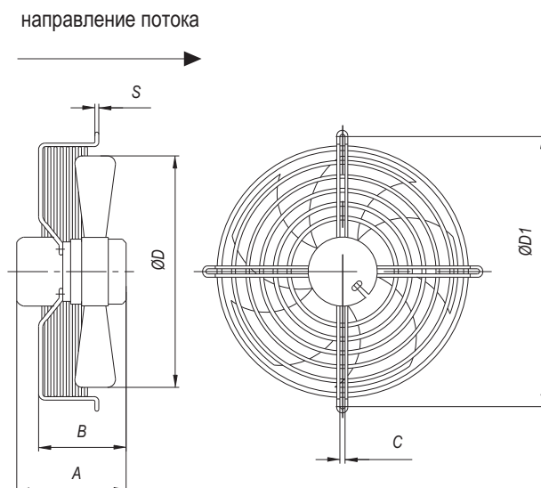
Габаритные размеры Вентиляторов VKVO
