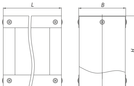
Пластиначатый шумоглушитель без обтекателя
