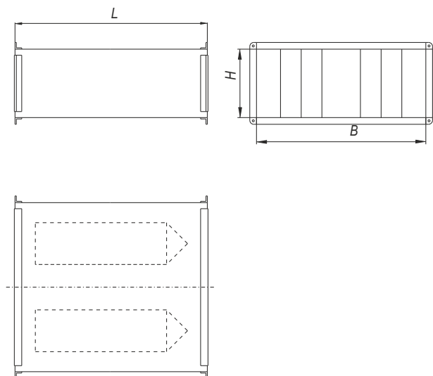
Пластиначатый шумоглушитель с обтекателем
