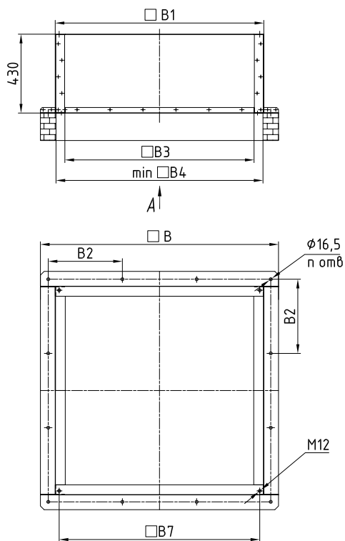
Стакан STKB-M
