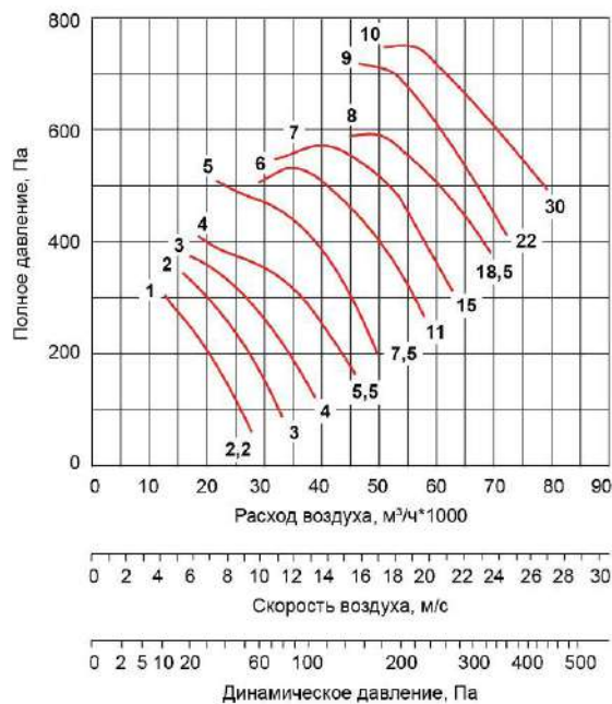
ВО-100-ДУ-.../1500-...
