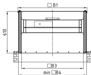
Стакан СТКВ-М
