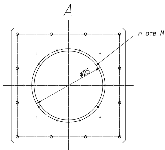
Стакан СКУ...- вид снизу
