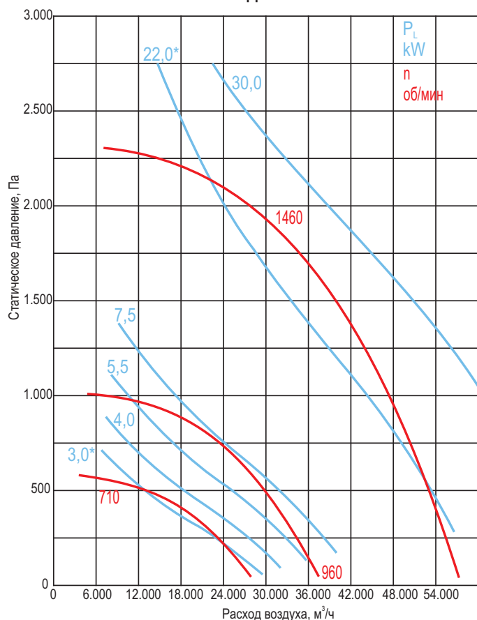
ВКР-9-ДУ-В-...
