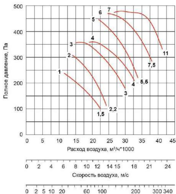
ВО-080-ДУ-.../1500-...
