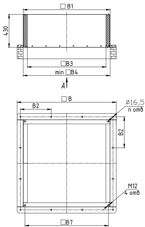
Стакан STKY-M
