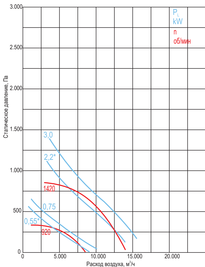
ВКР-5,6-ДУ-В-...
