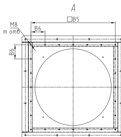
Стакан СТК... вид снизу
