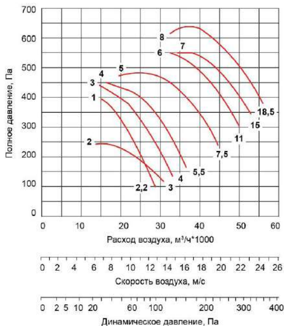
ВО-090-ДУ-.../1500-...
