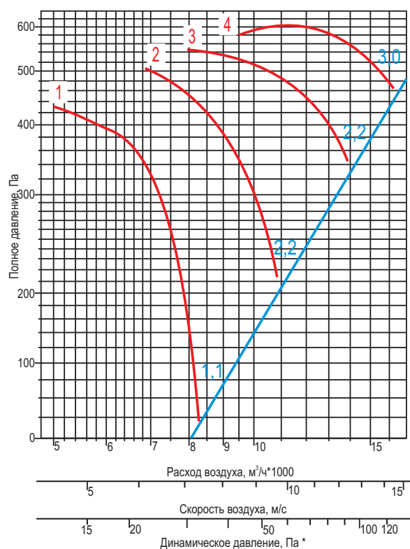
ВО 30-160-063
