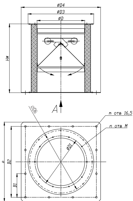
Стакан СКУ-П02 приток
