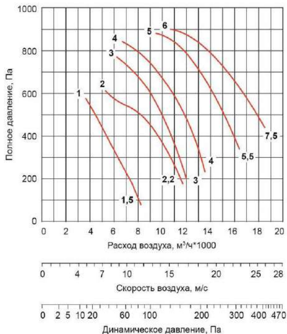
ВО-050-ДУ-.../3000-...
