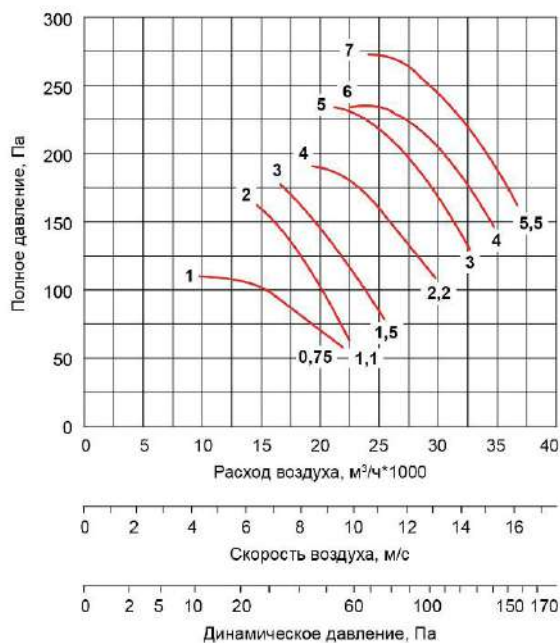
ВО-090-ДУ-.../1000-...
