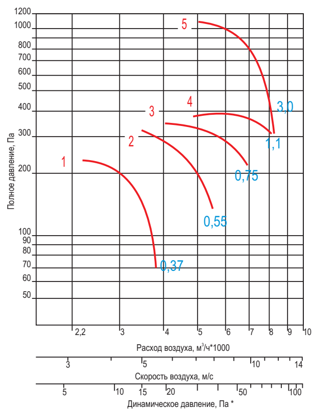
ВО 30-160-050
