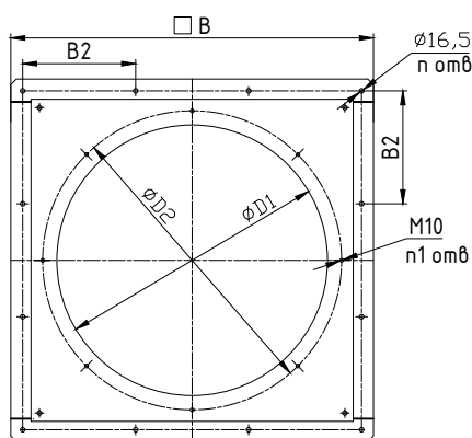
Стакан СТКУ-М
