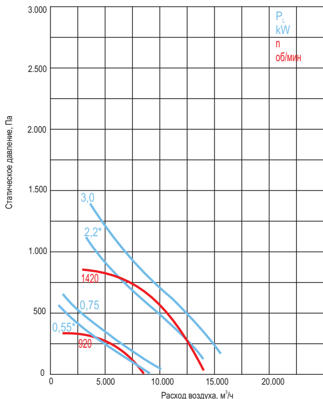
ВКР-5,6-ДУ-Ф-...
