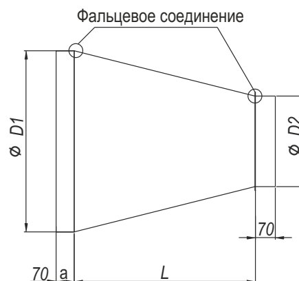
Переход с круглого на круглое сечение
