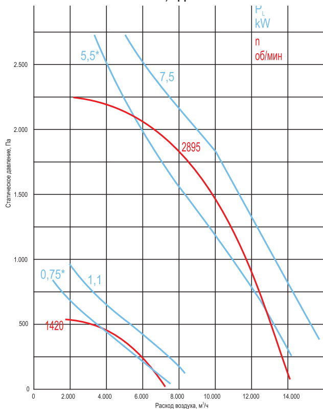
ВКР-4,5-ДУ-В-...
