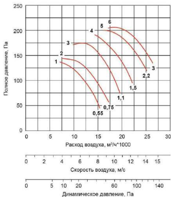
ВО-080-ДУ-.../1000-...
