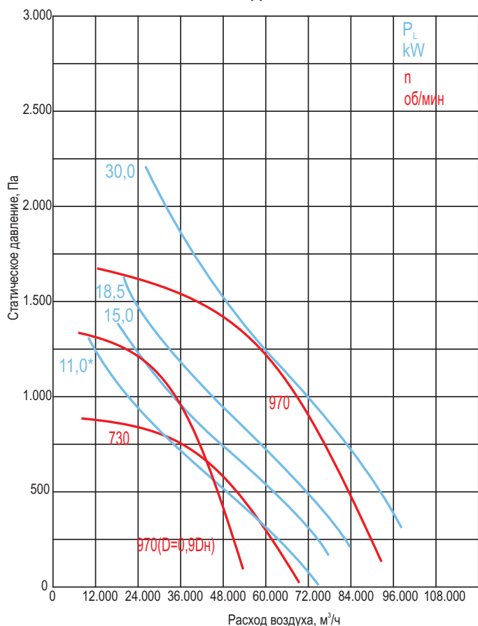
ВКР-11-ДУ-В-...
