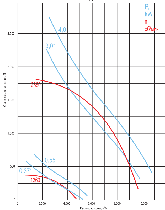
ВКР-5-ДУ-В-...
