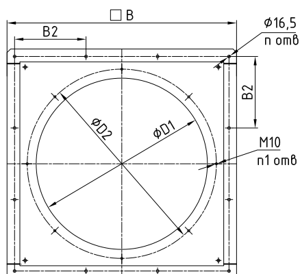
Стакан СТКВ-М
