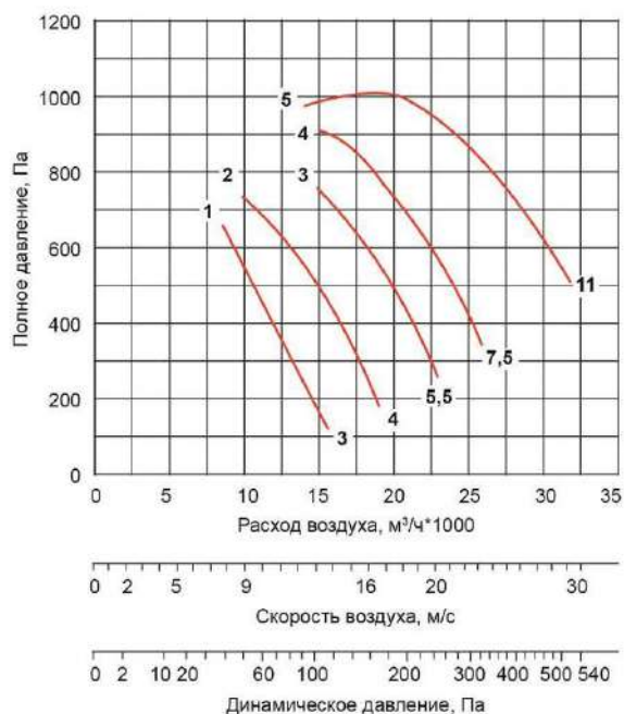
ВО-071-ДУ-.../1500-...
