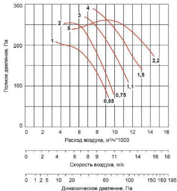
ВО-056-ДУ-.../1500-...
