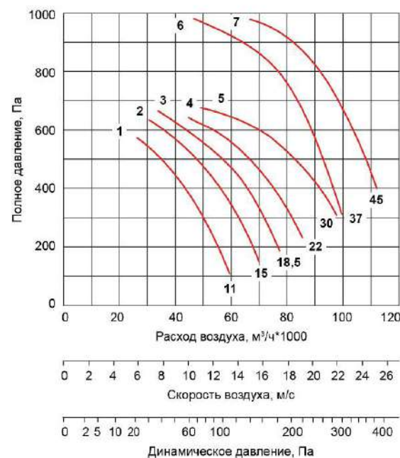
ВО-125-ДУ-.../1500-...
