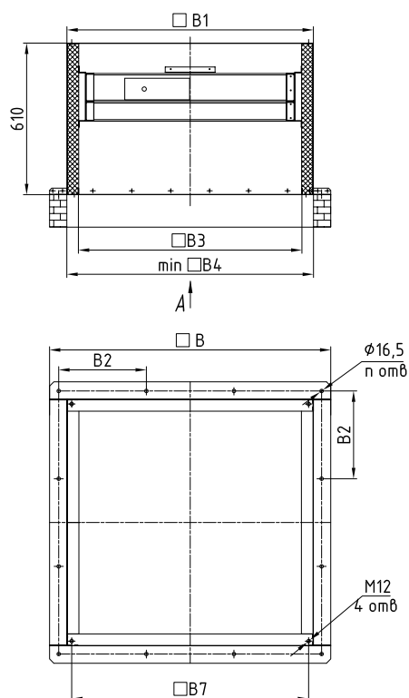
Стакан STKY-P
