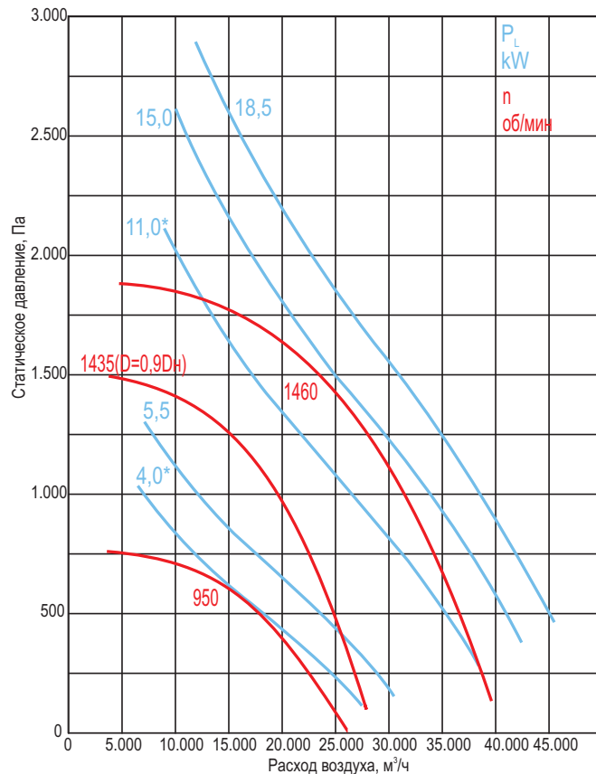
ВКР-8-ДУ-В-...
