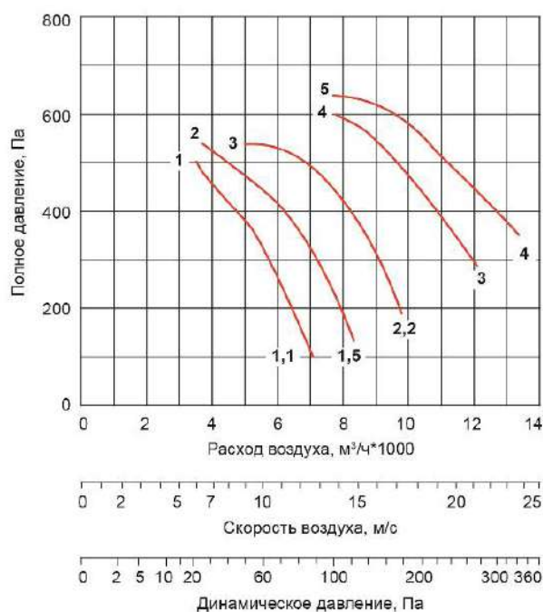
ВО-045-ДУ-.../3000-...
