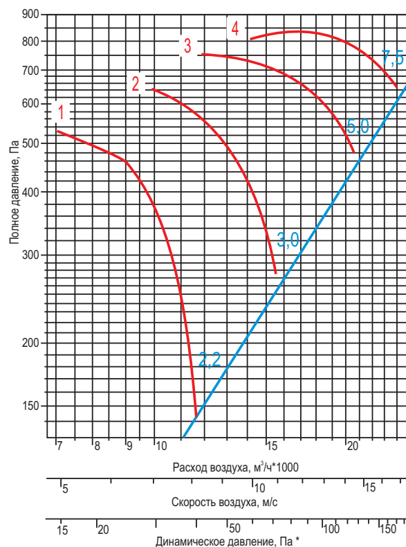
ВО 30-160-071
