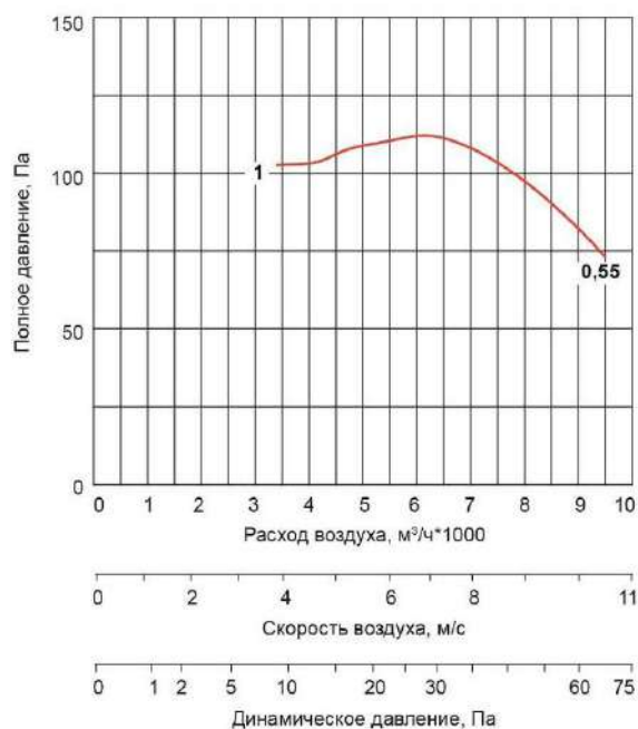
ВО-056-ДУ-.../3000-...
