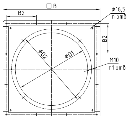
Стакан СТКУ-П
