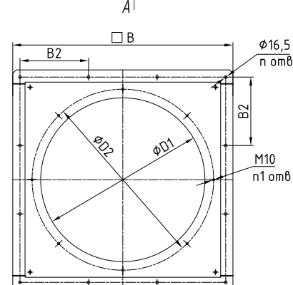
Стакан СТКУ-К
