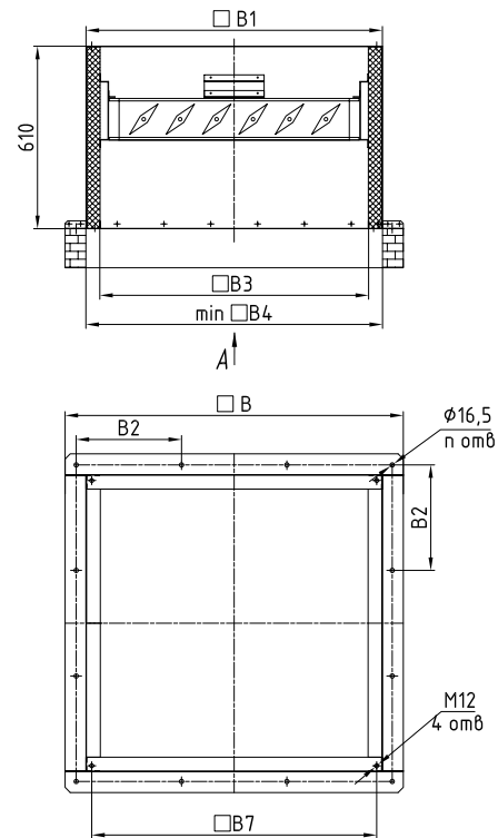
Стакан STKY-K
