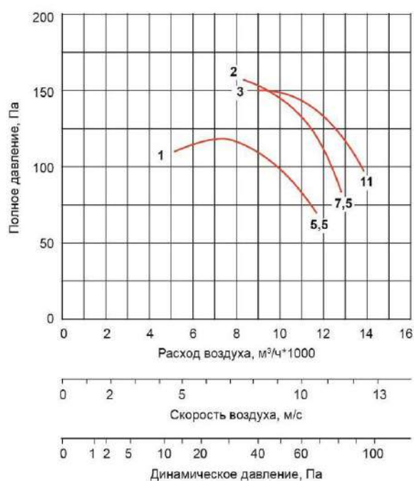
ВО-063-ДУ-.../1000-...
