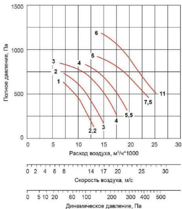
ВО-056-ДУ-.../3000-...
